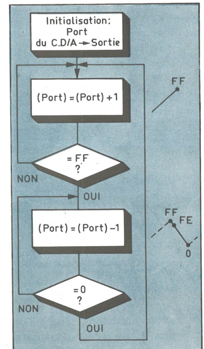
Fig. 9. - Organigramme de génération d'un signal triangulaire.
