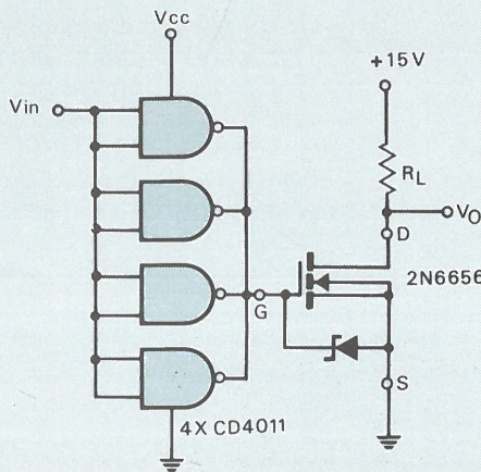
Fig. 11. - Commutateur rapide compatible CMOS.
