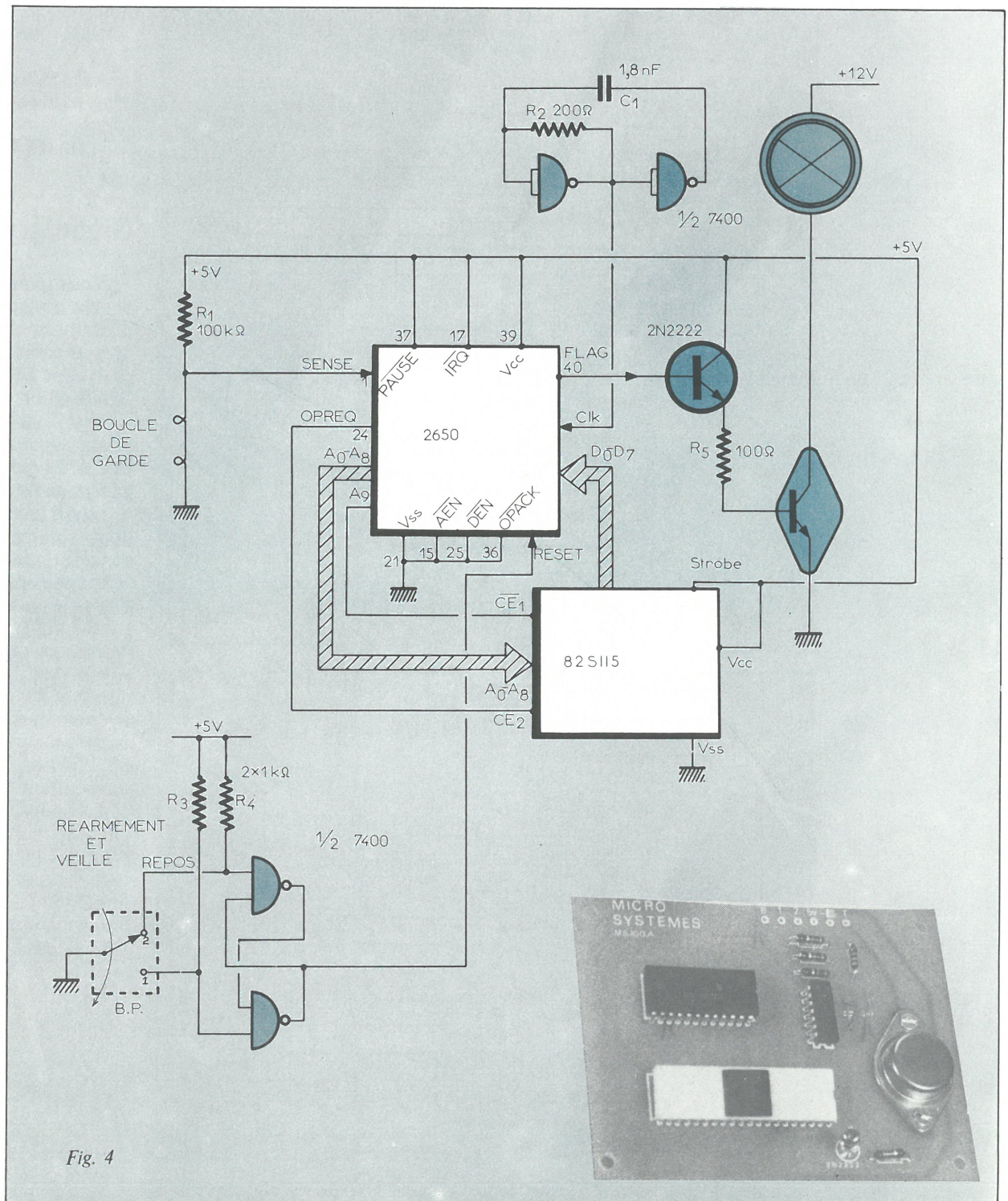
Fig. 4. - Schéma de fonctionnement. Le transistor de puissance peut être un 2N3055 ou équivalent. Sur le circuit imprimé câblé, on distingue aisément le microprocesseur (blanc), la mémoire PROM et le 7400 (vertical).
