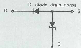
Fig. 8. - Circuit équivalent à l'état OFF ( V_{GS} = 0 ).
