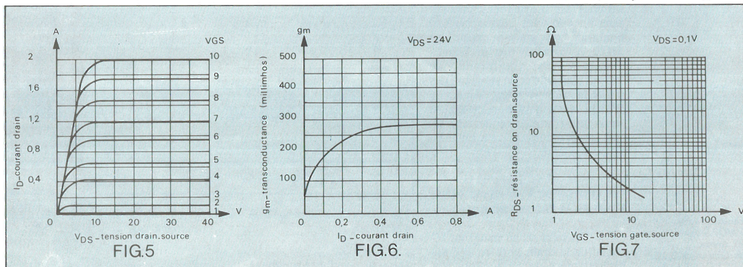
Fig. 7. - Caractéristique de la résistance drain-source en fonction de V_{GS} .
