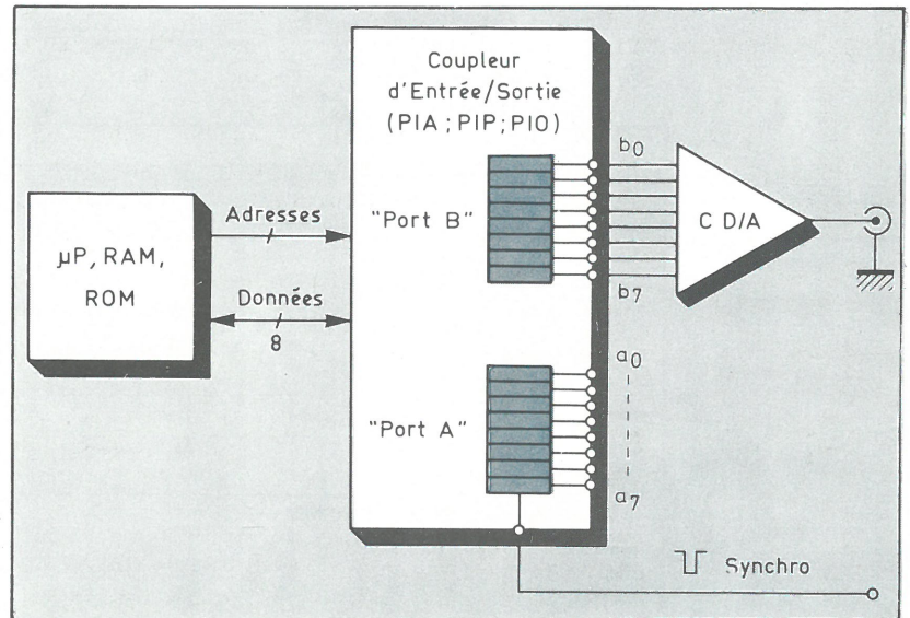
Fig. 4. - Le coupleur d'entrée/sortie est programmé en sortie. Le mot mémoire ou port B est relié bit à bit au convertisseur digital/analogique.
