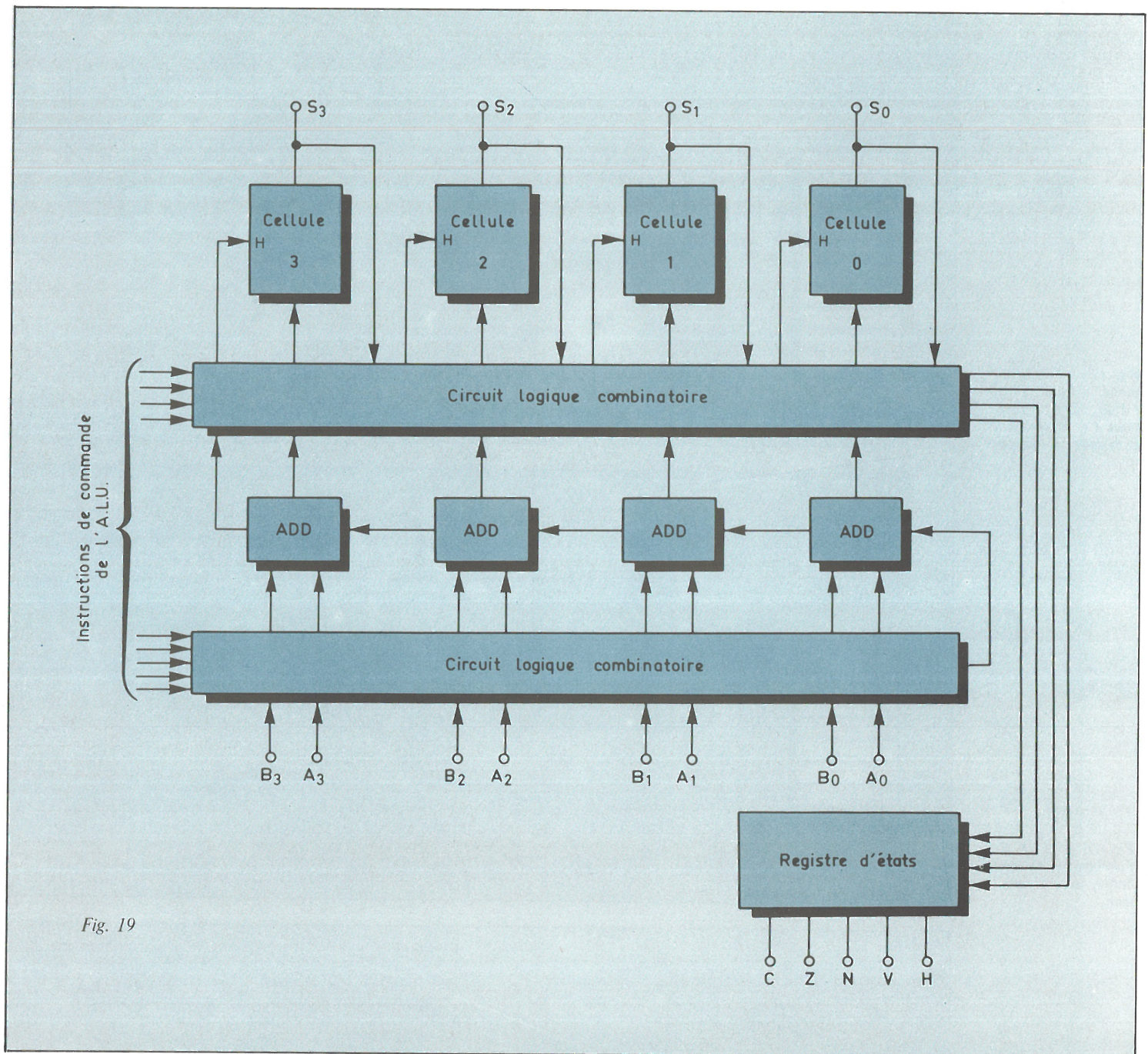
Fig. 19. - Schéma synoptique de l'ALU d'un microprocesseur.
