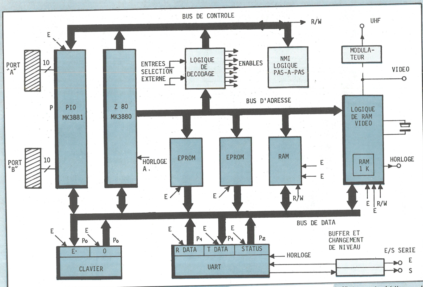
Fig. 1. - Le NASCOM 1 est organisé autour du Z80.
