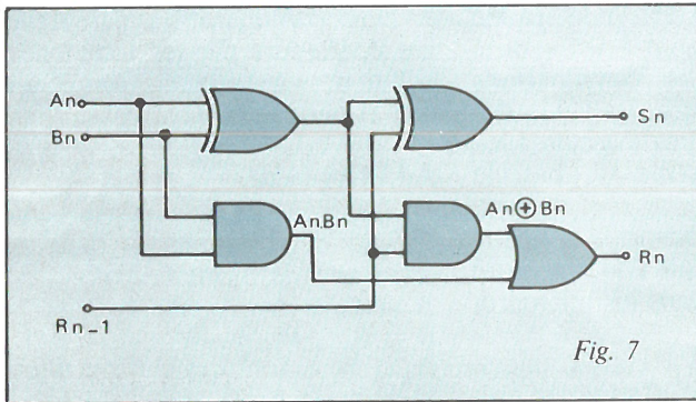
Fig. 7. - Principe d'un additionneur binaire.
