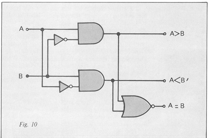
Fig. 10. - Comparateur : La fonction A = B est définie par A \oplus B . La fonction A > B est définie par A \bar{B} . La fonction A < B est définie par \bar{A} B .
