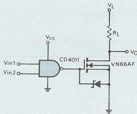
Fig. 10. - Commande d'un VN 66 AF par une porte CMOS.
