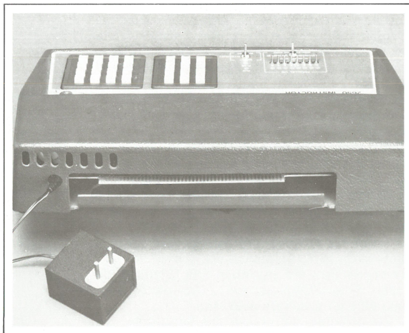
L'I 50 vue par sa face arrière. On aperçoit le circuit imprimé avec son BUS S 100. Au premier plan, le transformateur d'alimentation.
