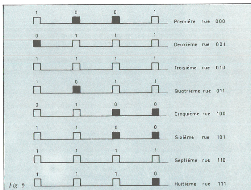
Fig. 6. - Huit rues parallèles de 4 maisons dont les lumières peuvent être allumées (« 1 ») ou éteintes (« 0 »), constituent un exemple d'une organisation mémoire de 8 mots de 4 bits.
