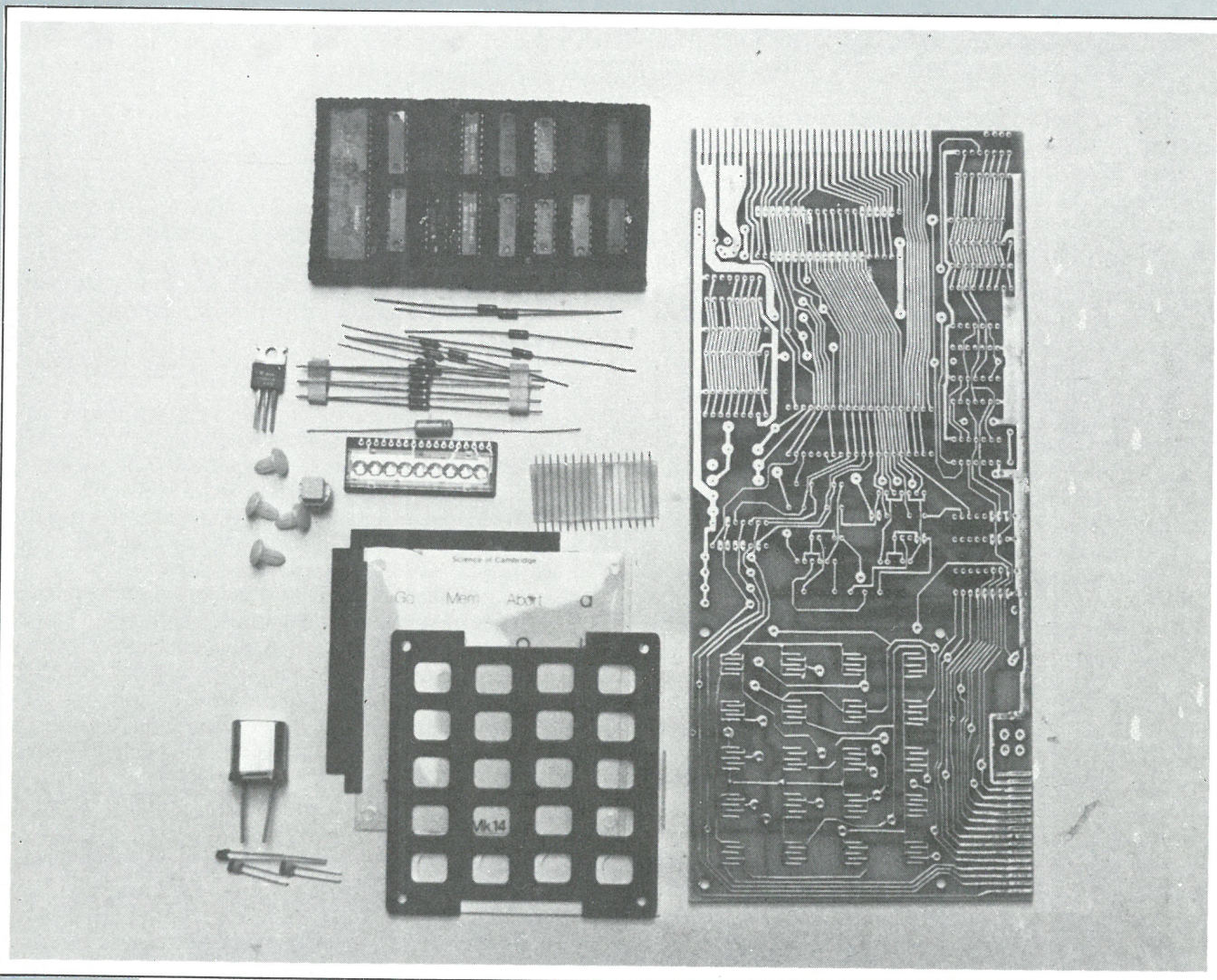
Le MK 14 : un kit d'initiation faible coût.
