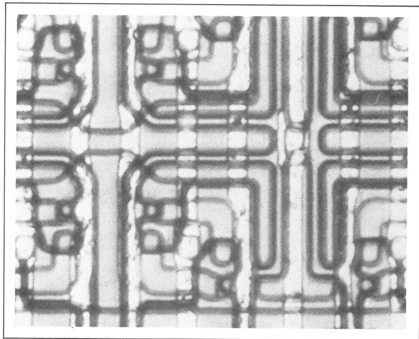
Cette microphotographie montre une mémoire RAM statique de 4 096 bits. La longueur du canal de chaque transistor MOS est de 4\mu\text{m} .
