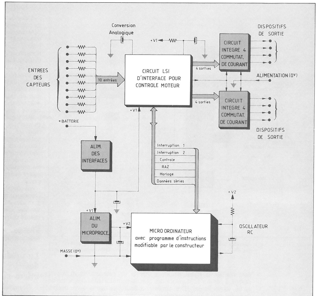
Fig. 3. - Système de contrôle total de moteur.
