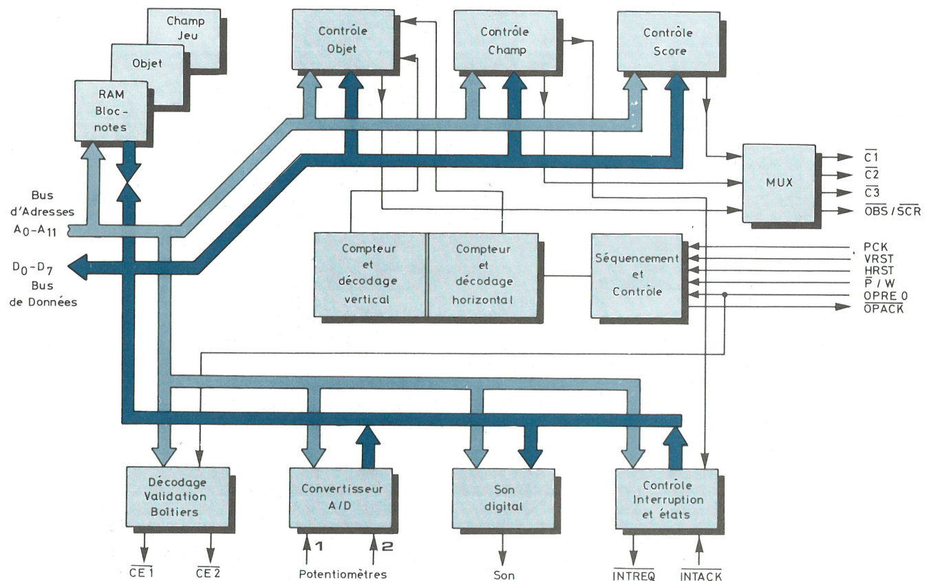
Fig. 3. - Architecture de l'interface vidéo programmable (PVI).
