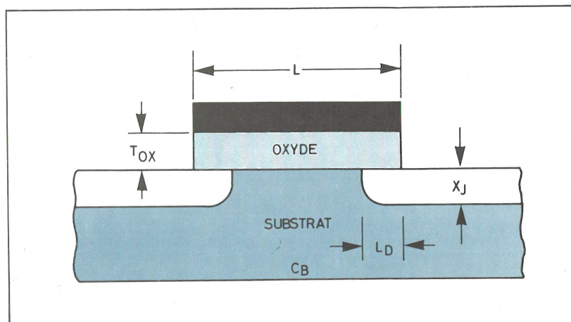
Fig. 1. - Pour réduire la taille d'un élément MOS, tous les paramètres physiques doivent être réduits proportionnellement. Si la longueur L du canal est multipliée par 1/S où S est le facteur de réduction, alors, l'épaisseur d'oxyde T_{ox} , la sous-diffusion latérale L_D , et la profondeur de jonction X_J doivent également être réduits par un facteur de 1/S . Dans le même temps, la constante de dopage du substrat C_B doit être multipliée par S .
