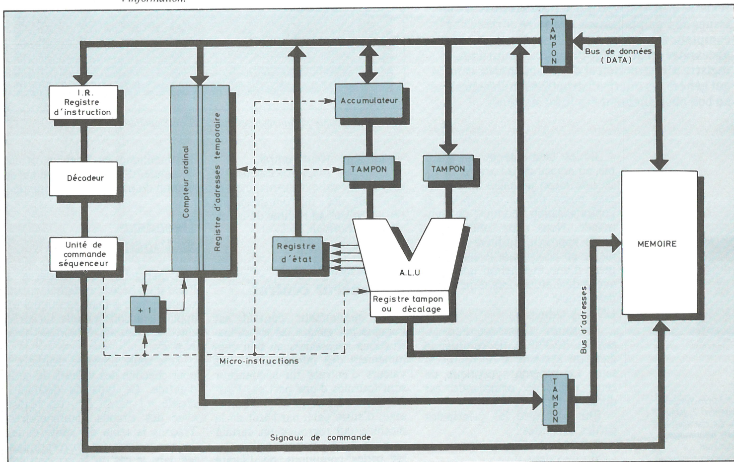
Fig. 1. - Emplacement de l'unité de commande dans un système de traitement de l'information.
