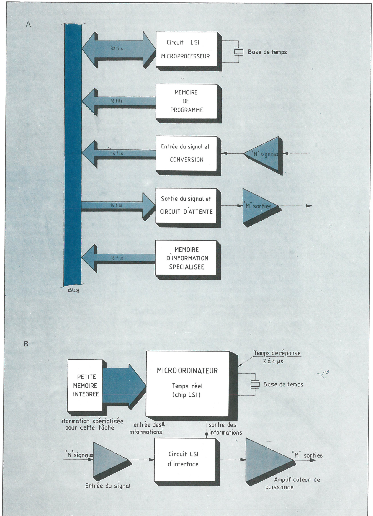
Fig. 2. - Deux approches possibles de la gestion d'un moteur d'automobile : un micro-ordinateur universel organisé autour d'un BUS (A) permet d'adapter le système à un grand nombre de fonctions ; un micro-ordinateur spécifique (B) réalise l'approche optimum d'un cas particulier.
