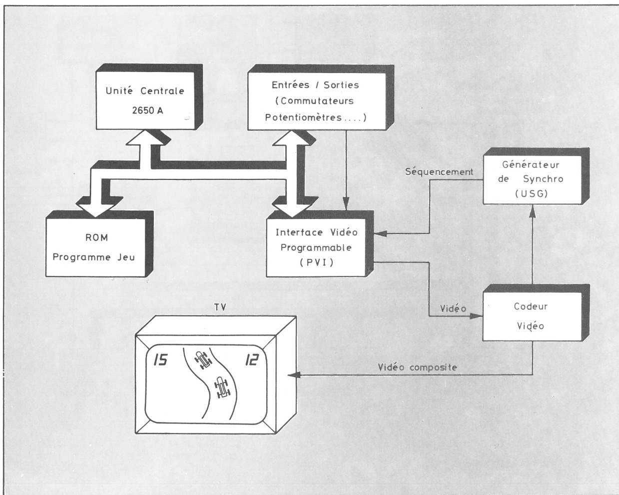
Fig. 2. - Jeu vidéo à microprocesseur : le concept « objet ». Ici, le microprocesseur lit le programme de jeu stocké en mémoire ROM et contrôle la vidéo présentée au récepteur T.V.
